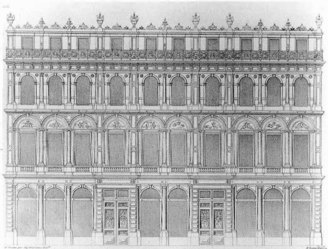
Opstand van de oorspronkelijke gevel van het huis van Jean-Pierre Cluysenaar, Kunstlaan 10 en 11.
